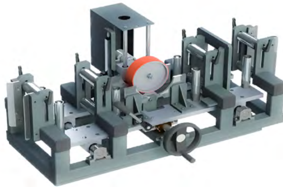
Abb. 1 MESSBOI 100 LC mit Vorwahlzähler im Gehäuse
